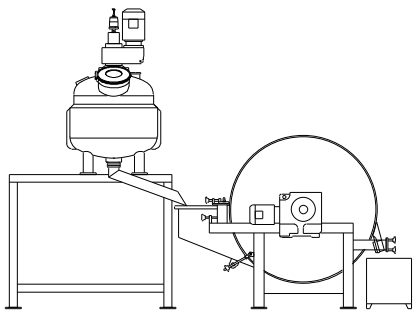
ELLB-800 PULLING MACHINE ELLB-800拉白机
